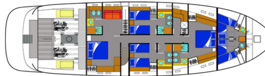
T85 Lowerdeck LUNGO RAGGIO
